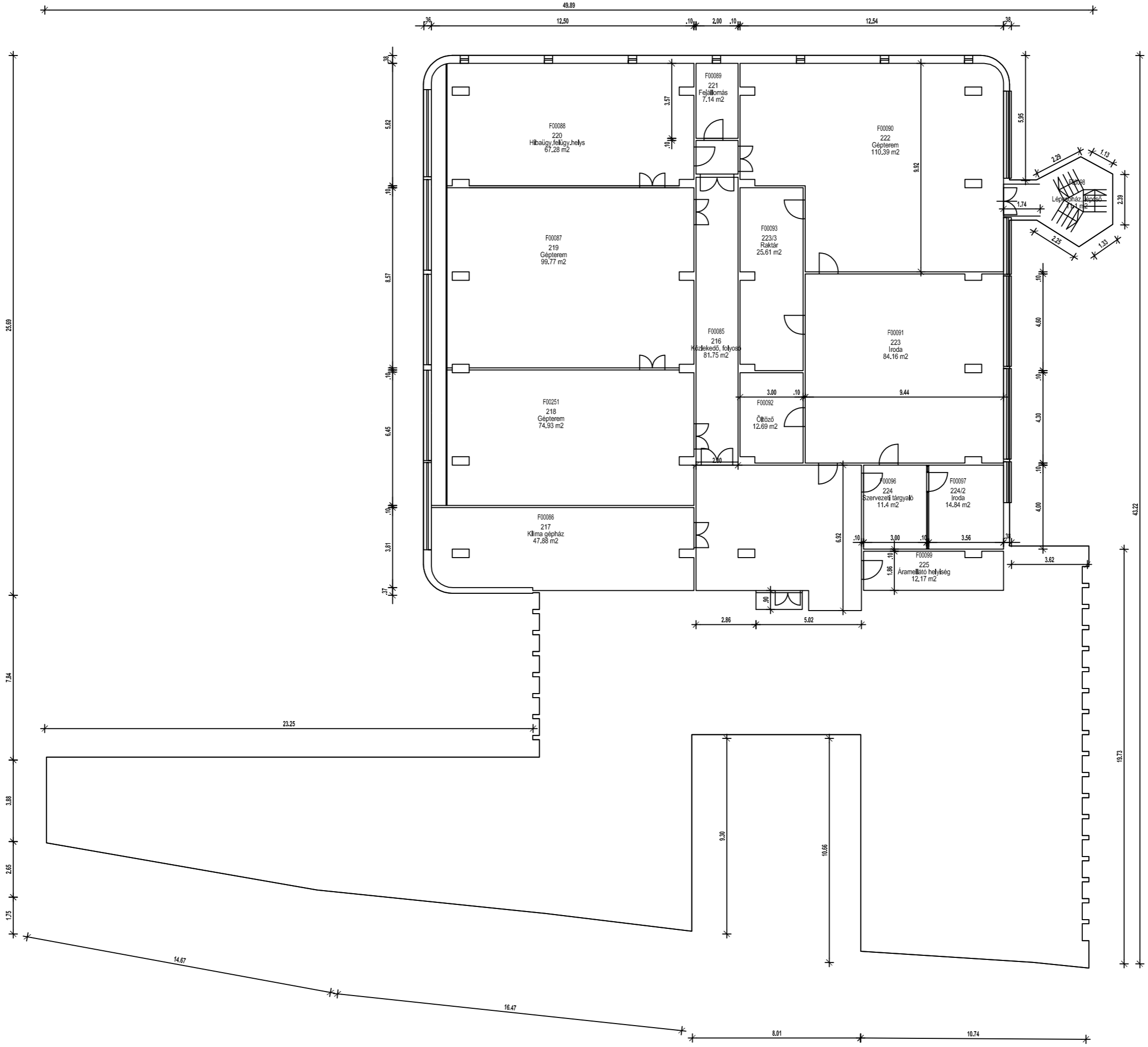
Budapest, József utca 19-23. Új épület - 2. Félemelet
